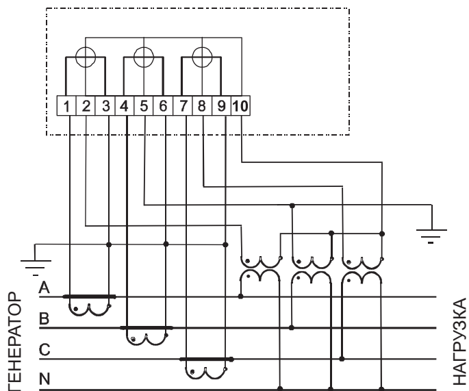
Рисунок Б.5 - Схема включения трехэлементного счетчика в четырехпроводную сеть с изолированной нейтралью и заземленной фазой В
