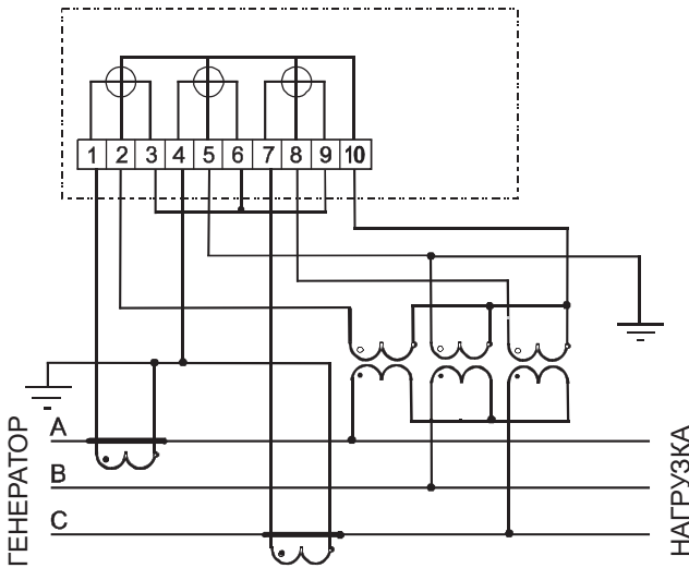
Рисунок Б.8 - Схема включения трехэлементного счетчика в трехпроводную сеть с тремя трансформаторами напряжения и заземленной фазой В
