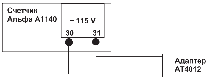
Рисунок Б.10 - Подключение к счетчику Альфа А1140 адаптера резервного питания
