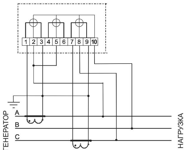
Рисунок Б.9 - Схема включения трехэлементного счетчика в трехпроводную сеть напряжением 0,22 кВ с изолированной нейтралью
