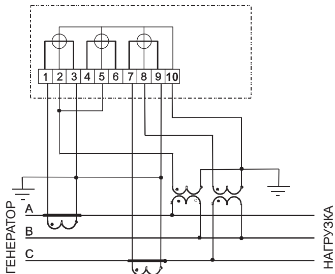
Рисунок Б.6 - Схема включения трехэлементного счетчика в трехпроводную сеть с двумя трансформаторами напряжения
