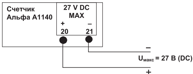
Рисунок Б.11 - Подключение импульсного выхода счетчика (при отсутствии дополнительного питания)
