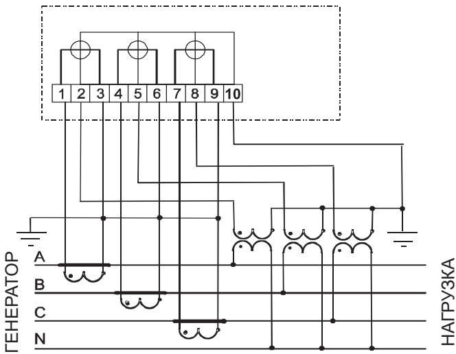
Рисунок Б.4 - Схема включения трехэлементного счетчика в четырехпроводную сеть с заземленной нейтралью
